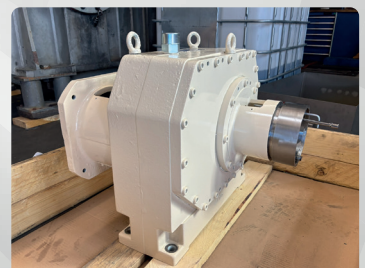
Extrudergetriebe im Auslieferungszustand Repariert von Nidec DESCH
